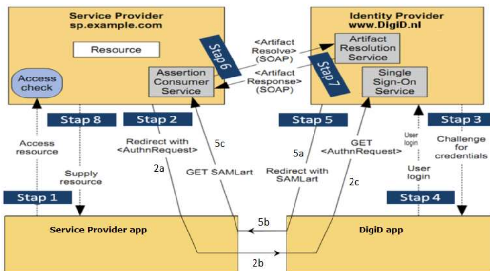
Figuur 3: SAML-authenticatiestappen voor app2app
