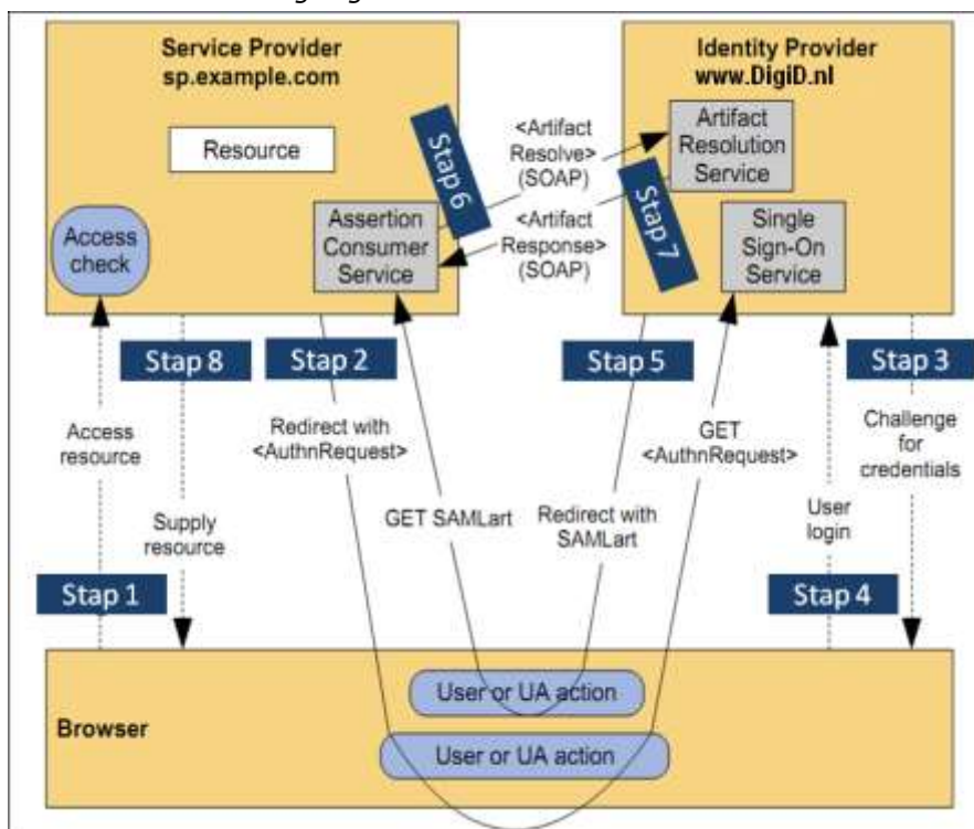
Figuur 1: SAML-authenticatiestappen
